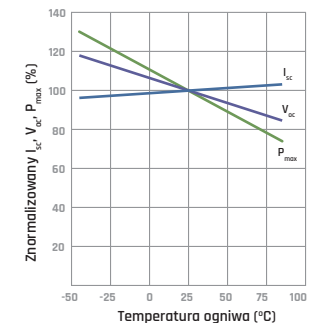
Osiągi w różnych warunkach temperaturowych
